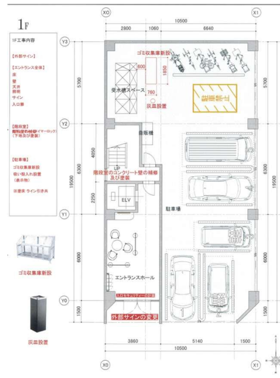
1階 平面図（予定）
